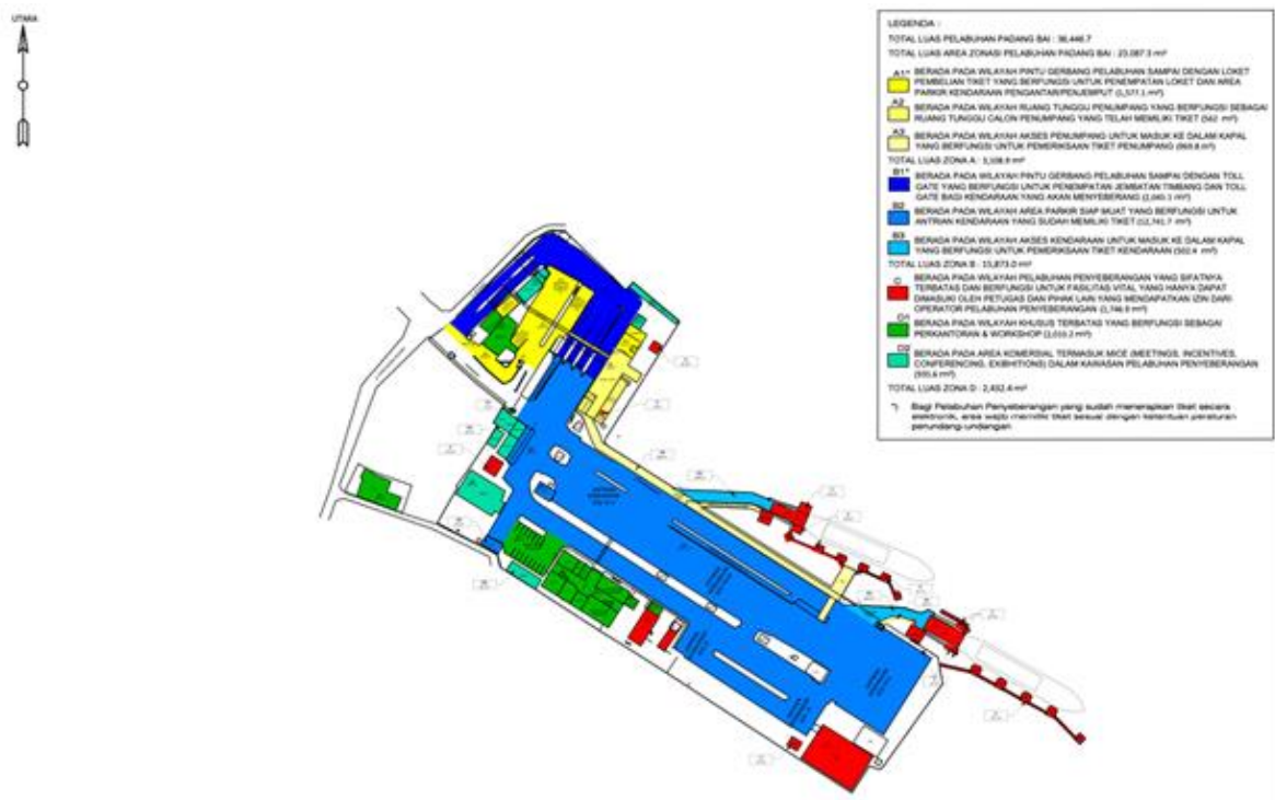
Gambar T.2.01 Layout Pelabuhan Padangbai
