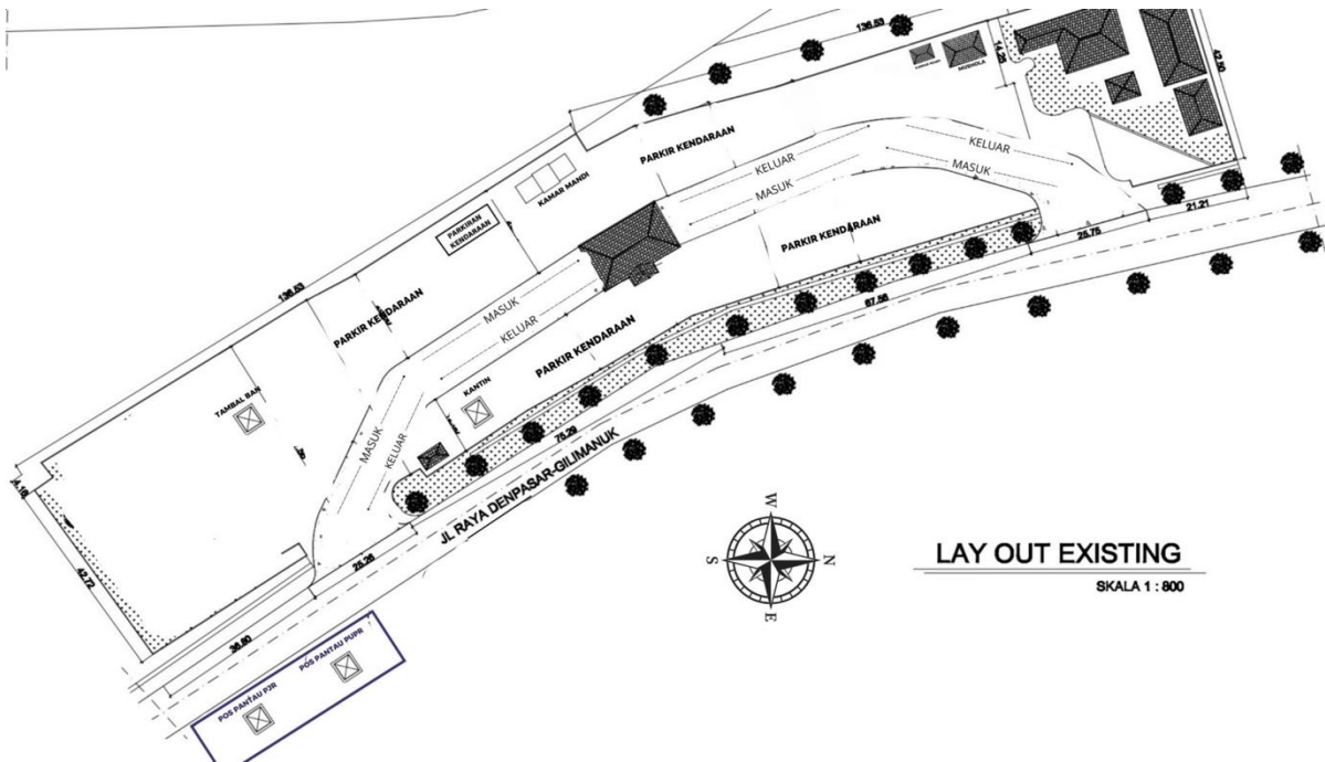
Gambar T.2.02 Layout UPPKB Cekik
