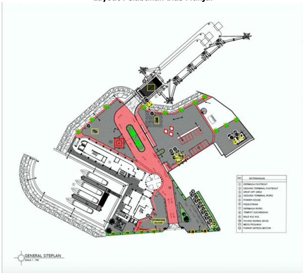
Gambar T.2.01 Layout Pelabuhan Bias Munjul
