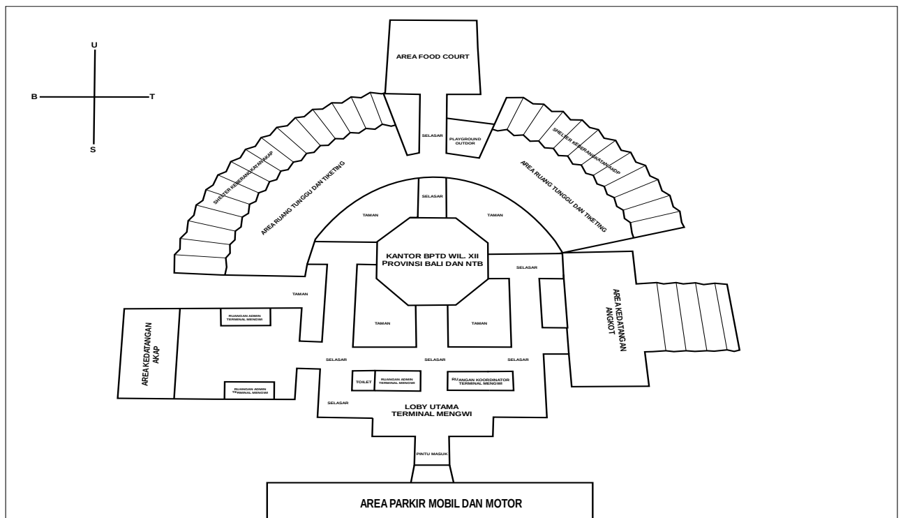
Gambar T.2.01 Layout Terminal Tipe A Mengwi
