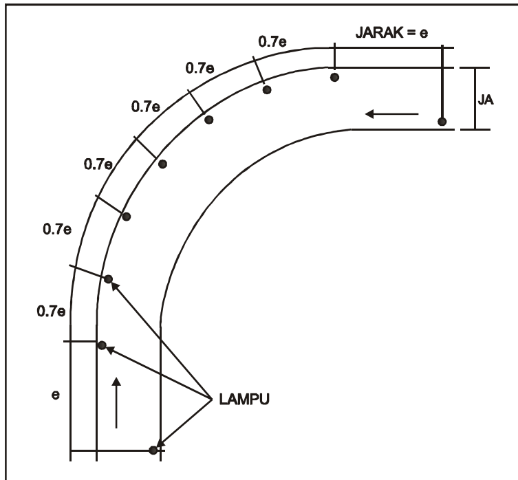
Gambar D.3 Lampu pada radius < 305\text{m} di lengkung luar
