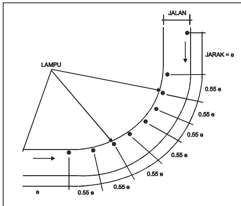
Gambar D.4 Lampu pada radius < 305\text{ m} di lengkung dalam
